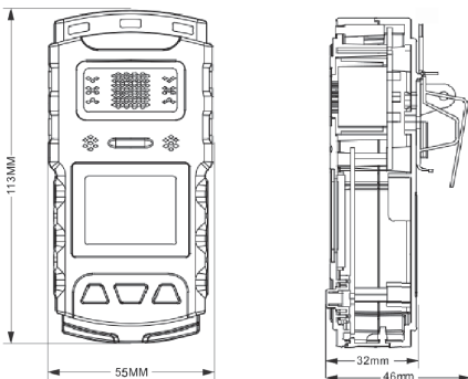
CTH1000 一氧化碳测定器外形尺寸
